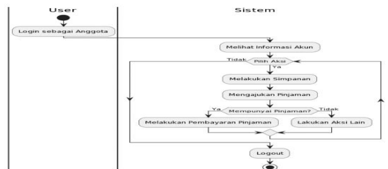
Gambar 9. Analisa sistem Yang Diusulkan
