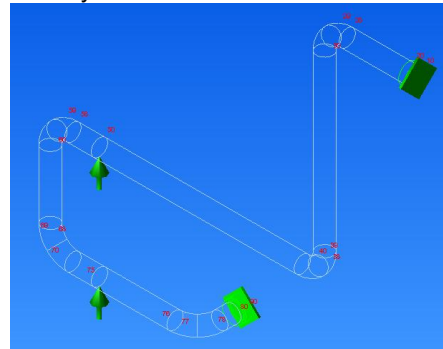
Gambar 4.7. Pemodelan pipa dan Node Referensi : Program CAESAR II 5.0
