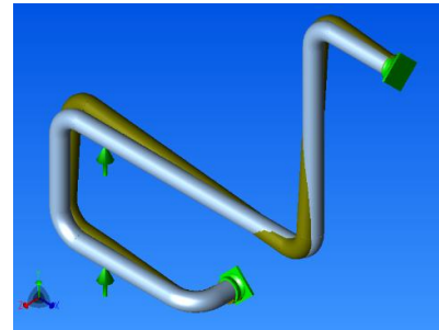
Gambar 4.6. Pemodelan pipa dengan expansi pipa
