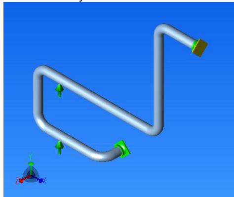
Gambar 4.5. Pemodelan pipa
