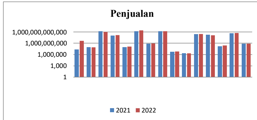
Gambar 2. Laporan Penjualan
