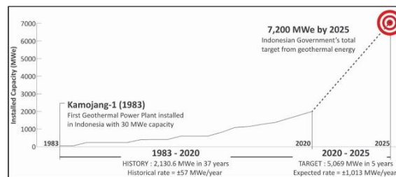
Gambar 1 Kapasitas dari pembangkit listrik tenaga panas bumi Indonesia yang terpasang dan target Pemerintah pada tahun 2025
