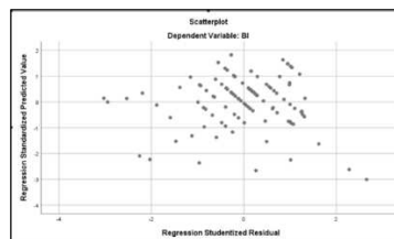
Gambar 16. Uji Heteroskedastisitas
