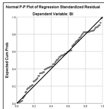
Gambar 15. Uji Normalitas
