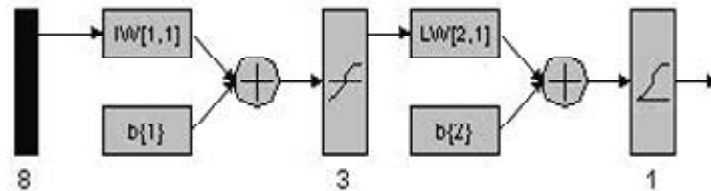
Gambar 8. Arsitektur BP2
