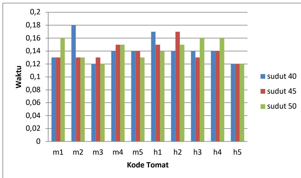
Gambar 9 Waktu jerit gripper
