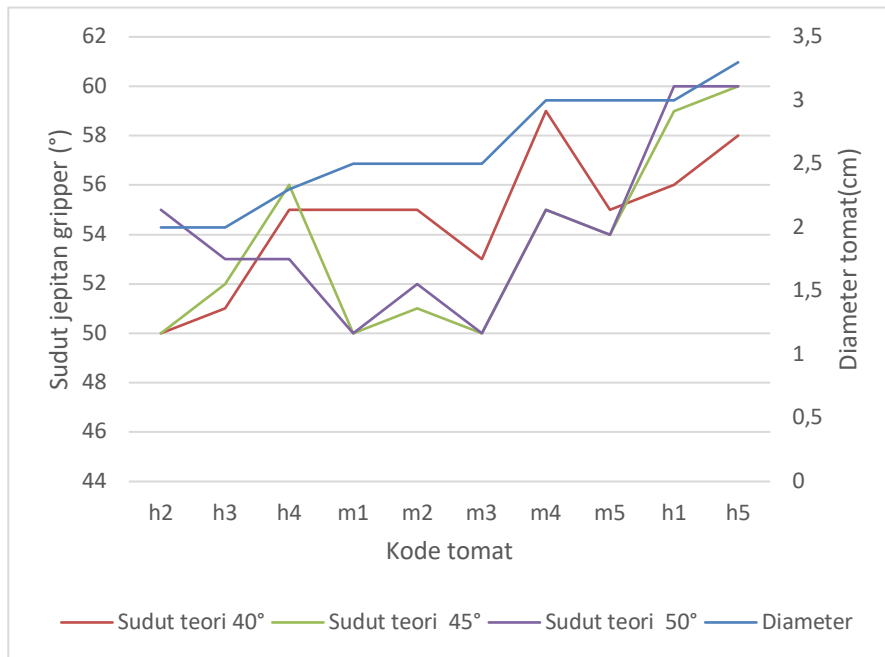
Gambar 6 Hubungan sudut jepitan dan diameter
