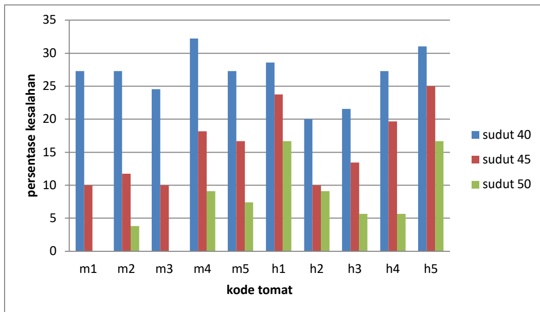
Gambar 7 Akurasi sudut jepit gripper
