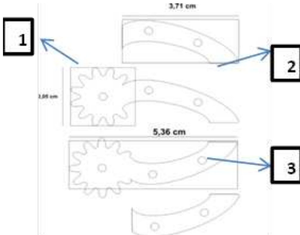
Gambar 2. Desain Gripper : (1) Gear gripper (penjepit); (2) Link gripper (penjepit) bagian atas; (3) Link gripper (penjepit) bagian bawah.
