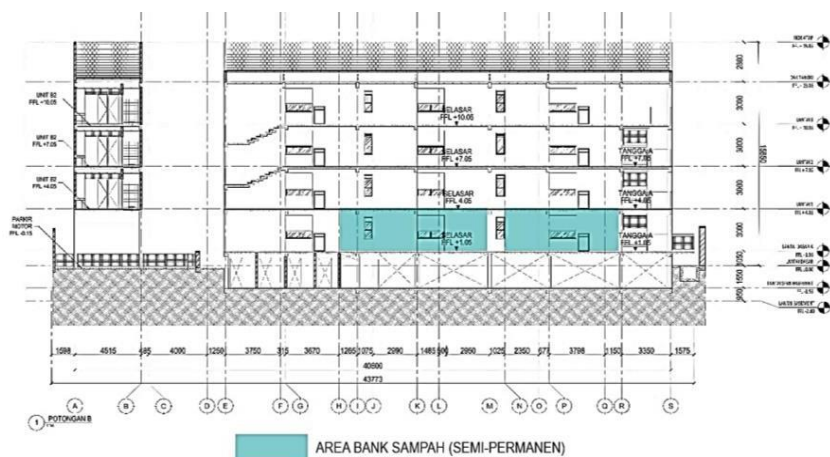
Gambar 10. Gambar Potongan B (Lokasi Area Bank Sampah)
