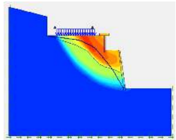
Gambar 13. Kondisi Setelah Terjadi Longsoran (SF = 1.1602)
