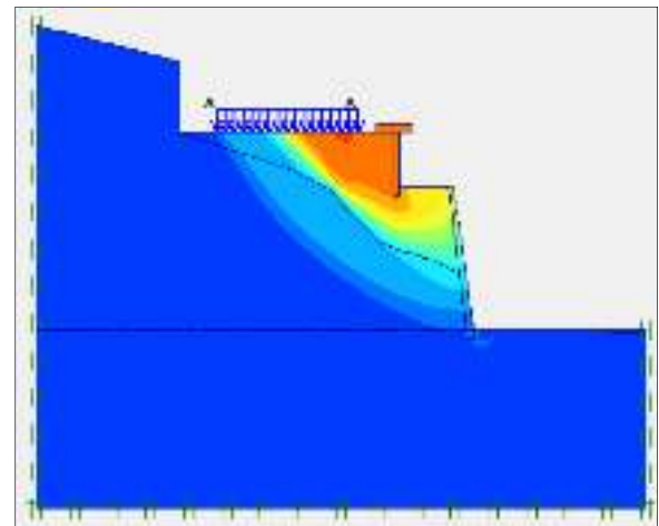
Gambar 12. Kondisi sebelum terjadi longsoran (SF = 1.3379)
