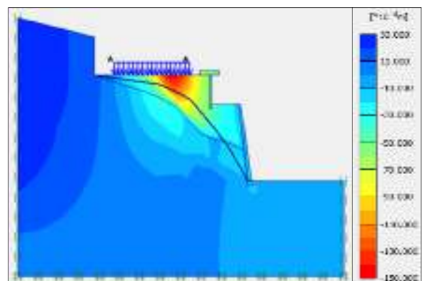
Gambar 11. Vertikal Displacement (Vertical disp.= 146.04 \times 10^{-3} m)
