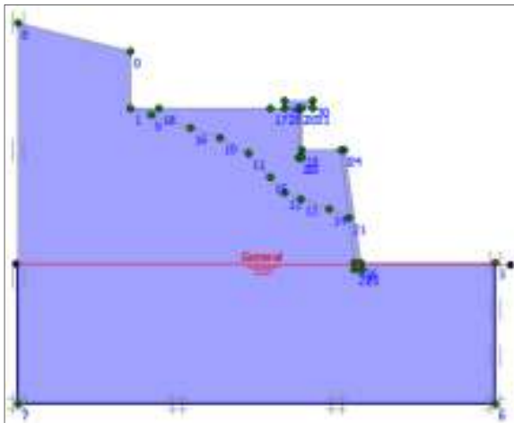
Gambar 4. Model Sebelum Terjadi Kenaikan Muka Air Tanah
