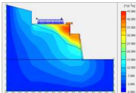
Gambar 8. Vertikal Displacement (Vertical disp.= 72.32 \times 10^{-3} m)
