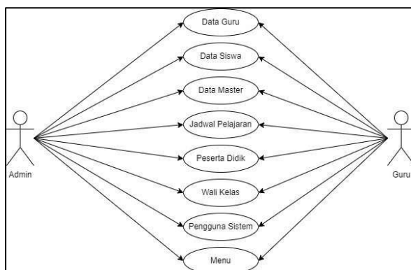
Gambar 2 Use Case Diagram Sistem Informasi Akademik
