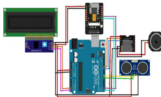
Gambar 1 Rangkaian Sistem
