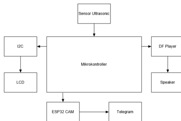
Gambar 2 Diagram blok desain konsep sistem.
