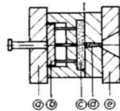
Gambar 2 cetakan Injection Molding [28].
