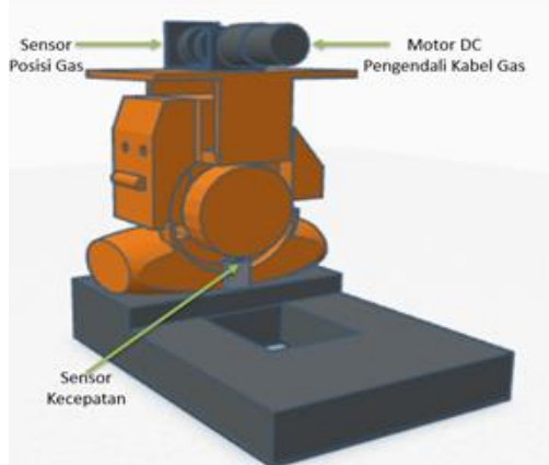
Gambar 4. Desain Alat
