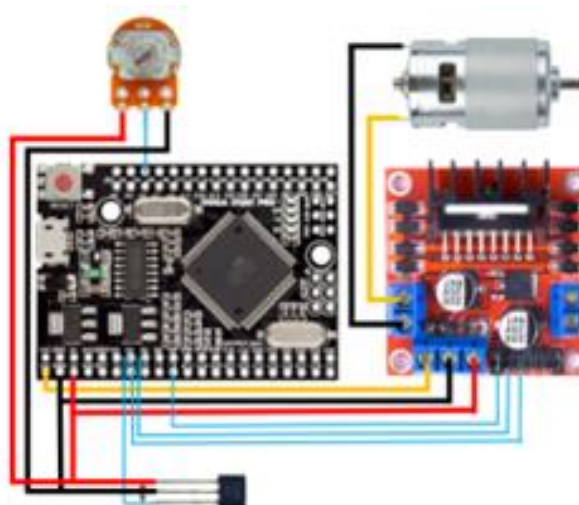
Gambar 3. Skema Rangkaian Alat
