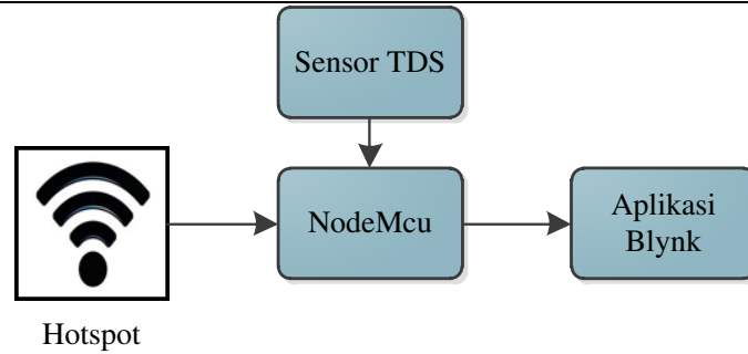
Gambar 2.1 Aristektur Pengiriman data dengan konsep IOT
