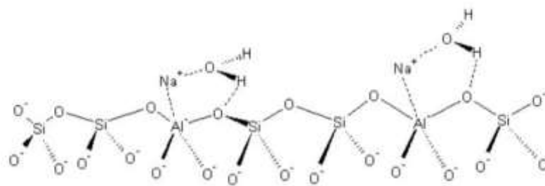
Gambar 3. Alumina dan Silika pada struktur zeolit
