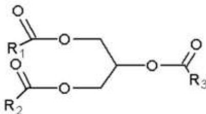
Gambar 2. (Ester dari asam lemak bebas), dimana R1, R2 dan R3 adalah rantai alkil dari asam-asam lemak.
