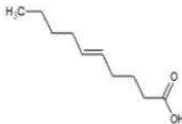
Gambar 5. Struktur asam lemak tak jenuh
