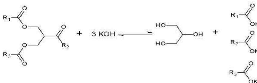
Gambar 8. Reaksi menyabunkan 1 g minyak dalam reaksi
