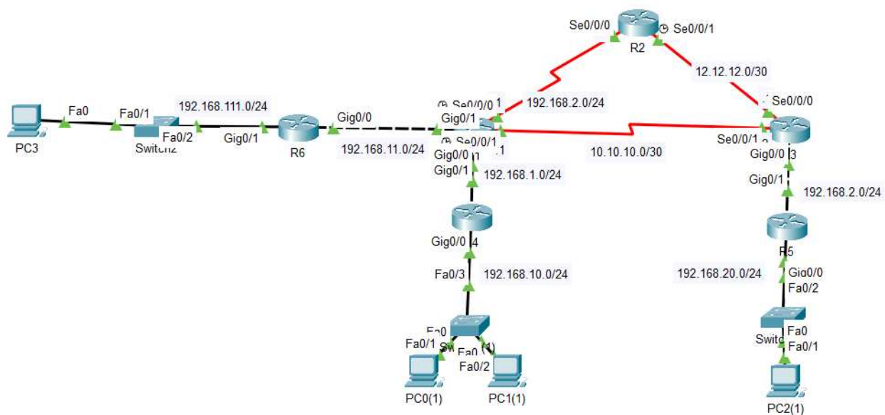
Gambar 1. Skema Jaringan
