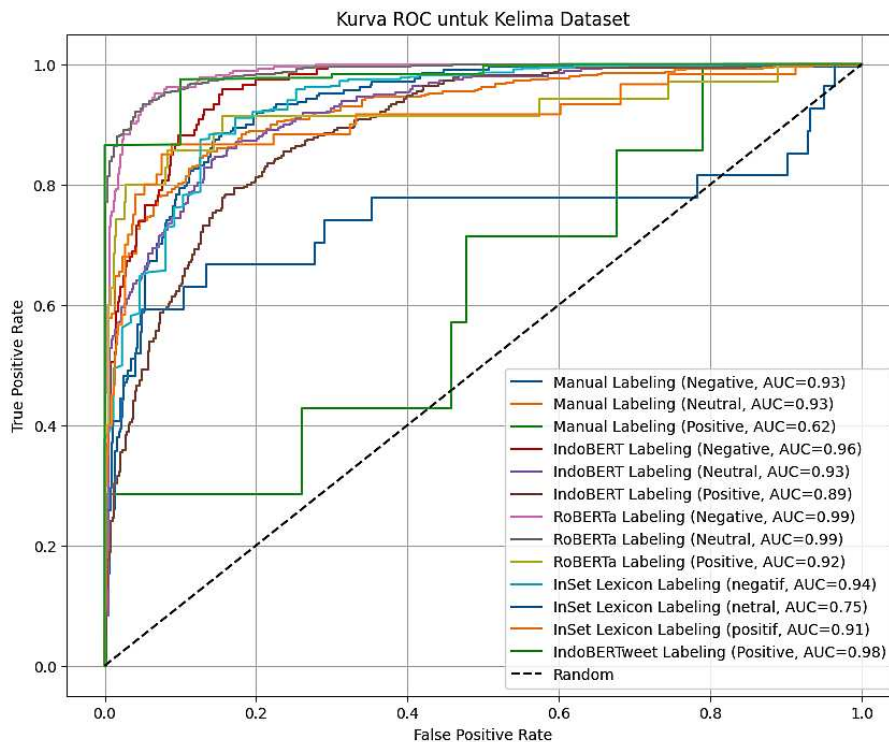
Gambar 3. Kurva ROC
