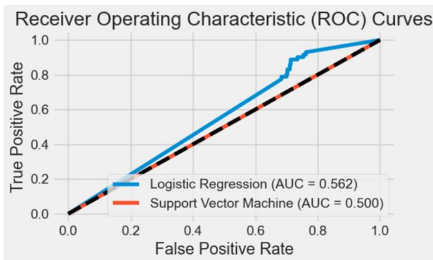
Gambar 13. Perbandingan kedua algoritma
