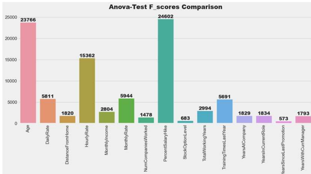
Gambar 6. Visualisasi F_score dari uji anova
