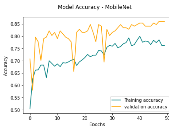
Gambar 4. Grafik akurasi saat training
