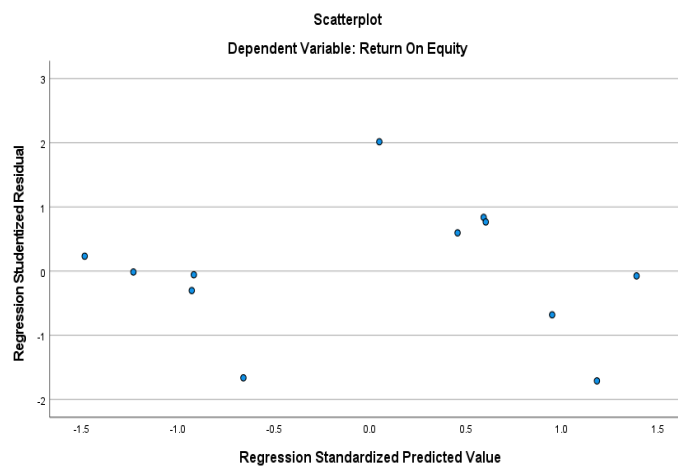
Gambar 2. Uji Heteroskedastisitas
