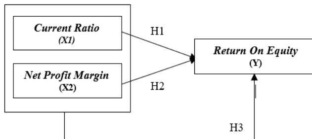
Gambar 1. Kerangka Berfikir
