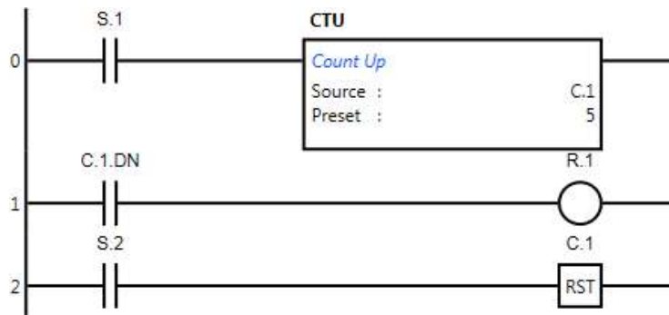
Gambar 2. Program Sistem Penghitung (Counter) dengan Software Outseal
