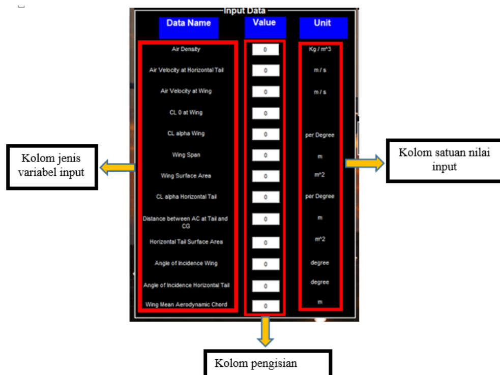
Gambar 4. Panel Input Data Aplikasi A-SSC
