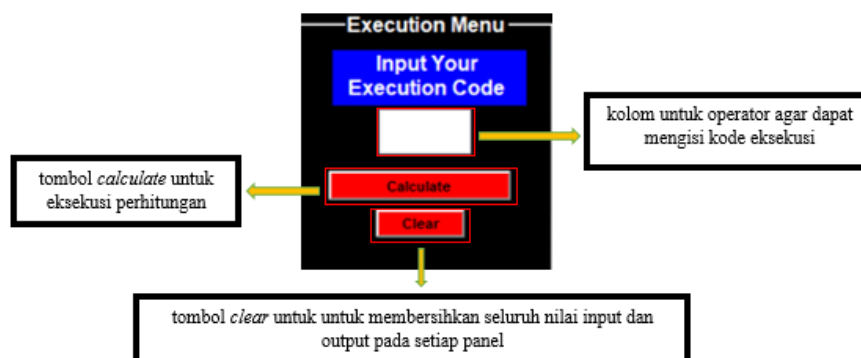
Gambar 7. Panel Execution Menu Aplikasi A-SSC
