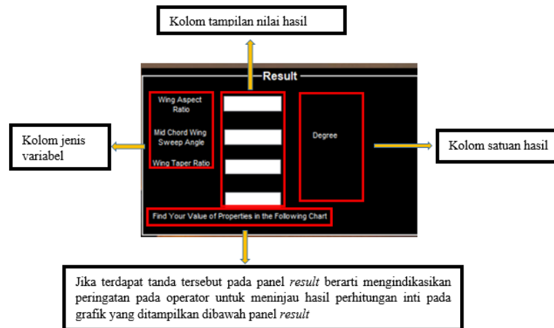
Gambar 8. Panel Result Aplikasi A-SSC
