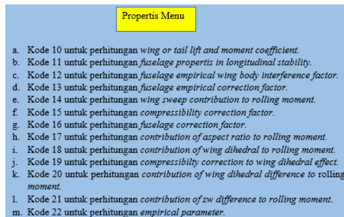
Gambar 6. Kode Eksekusi Untuk Menu Hitung Propertis Pada Aplikasi A-SSC
