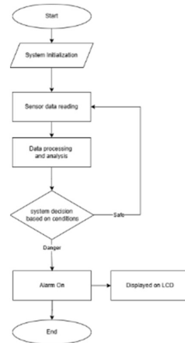
Gambar 4. Alur Kerja Sistem
