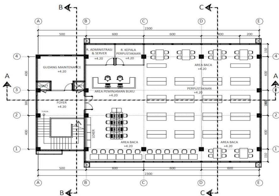
Gambar 4. Denah lantai 2 – Perpustakaan
