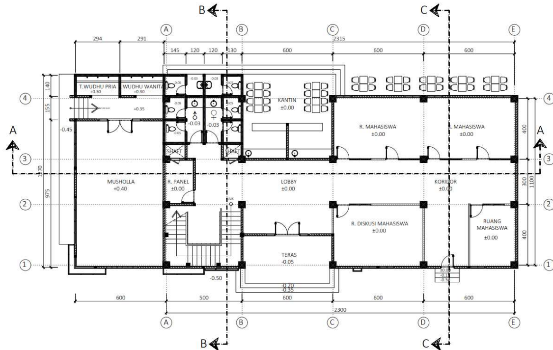
Gambar 3. Denah lantai 1 - Pusat Kegiatan Mahasiswa
