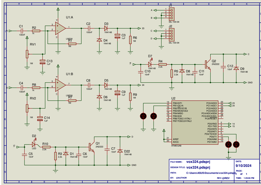
Gambar 9 Rangkaian lengkap interface
