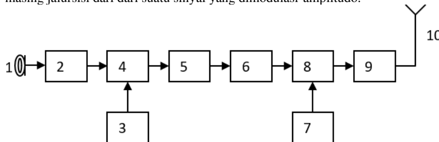
Gambar 4 Blok diagram pemancar SSB
