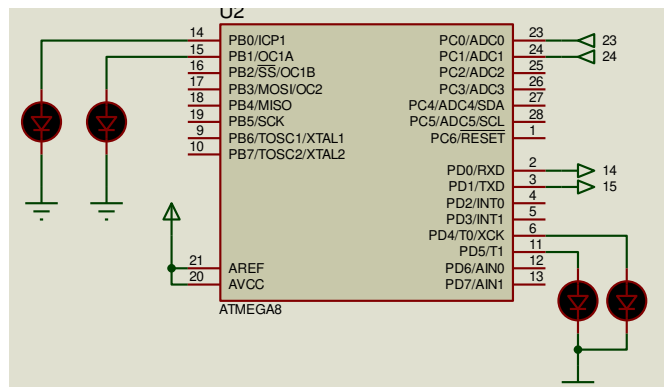
Gambar 10 Rangkaian untuk ATmega8
