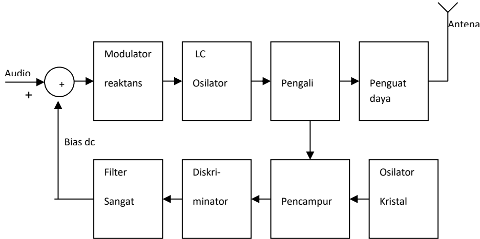
Gambar 2 Blok diagram pemancar FM
