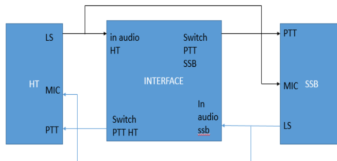
Gambar 7 Model sistem HT ke SSB dan SSB ke HT
