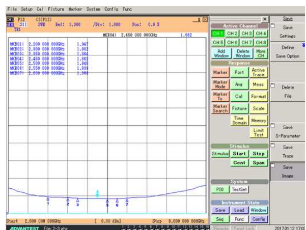
Gambar 5. Hasil Pengukuran VSWR
