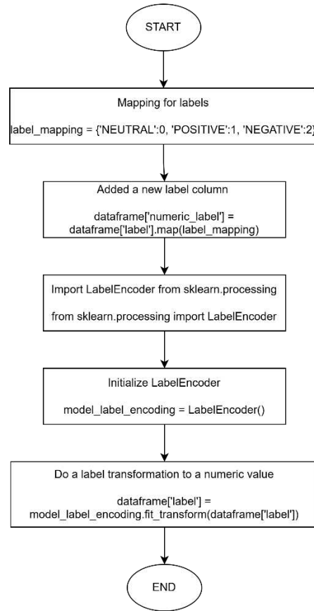
Fig. 3. Label Encoding
