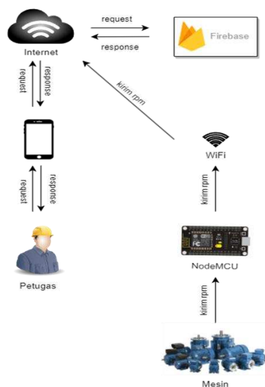
Gambar 2. Arsitektur Sistem
