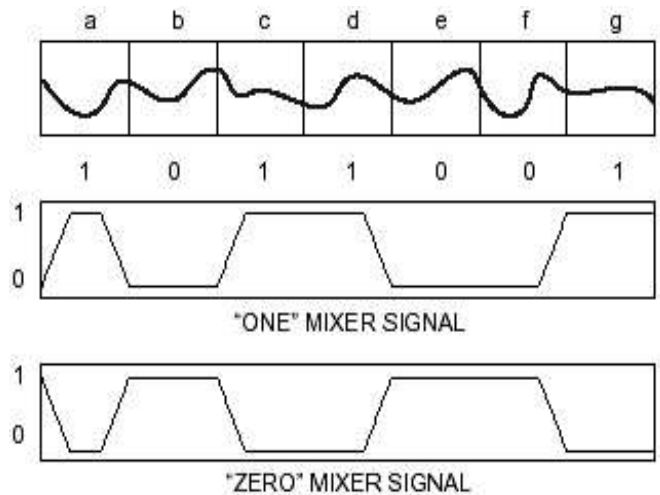
Gambar 4. Sinyal mixer
