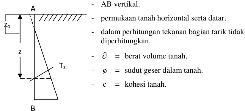
Gambar 1 Tekanan Tanah Lateral Horizontal
