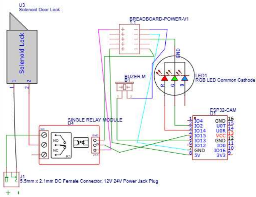
Gambar 4. Skema Rangkaian Perangkat Keras
