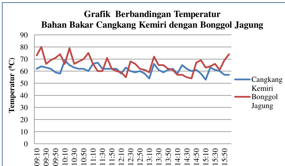
Gambar 8 Grafik perbandingan temperatur bahan bakar cangkang kemiri dengan bonggol jagung.
