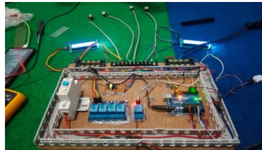
Gambar 7 Perakitan dan pengujian fungsi sistem kontrol Arduino Atmega328.
