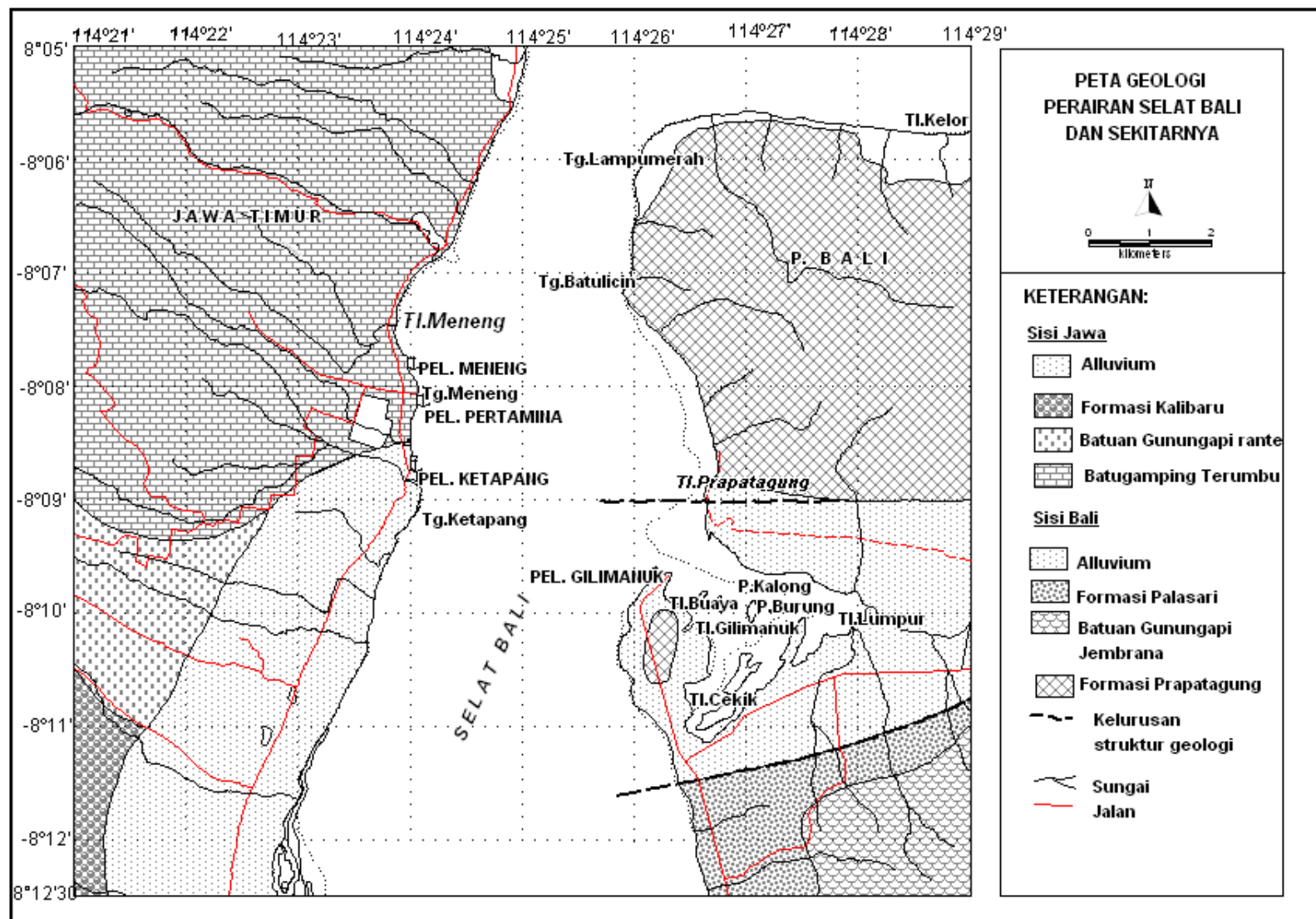
Gambar 2. Peta geologi perairan Selat Bali dan sekitarnya (Purbo Hadiwidjojo, 1974).
