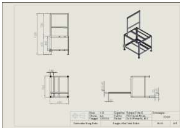
Gambar 2. Rancangan Rangka 2 dimensi
