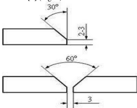
Fig. 3. Groove
