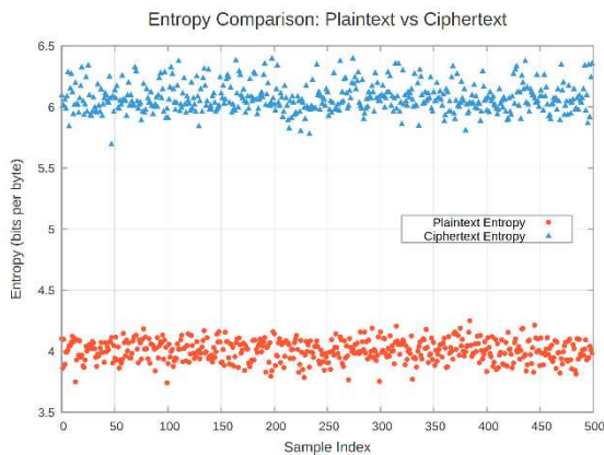
Gambar 6. Hasil Pengukuran Entropi.
