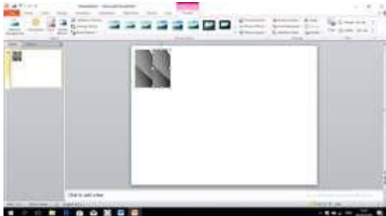
Gambar 14. Hasil Translasi
