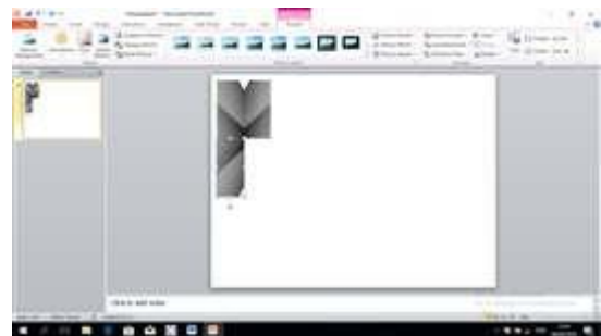
Gambar 17. Hasil Rotasi
