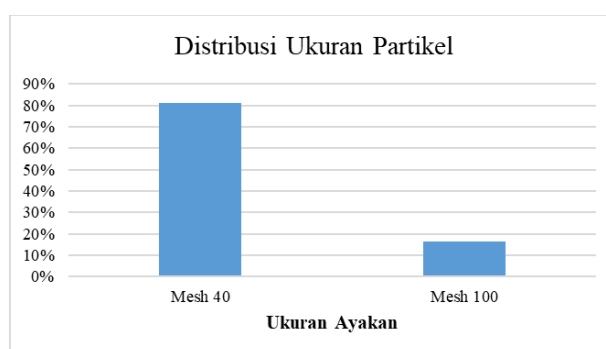
Gambar 4. Grafik Mikromeritik
