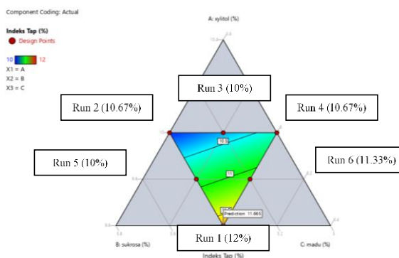
Gambar 3. Contour Plot Indeks Tap Granul Instan
