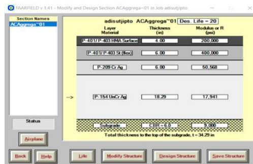
Gambar 4 Hasil Evaluasi Tebal Perkerasan Menggunakan Program FAARFIELD
