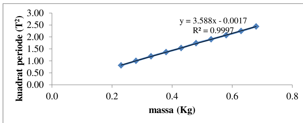
Gambar 10. Grafik hubungan antara massa dengan periode pegas 2
