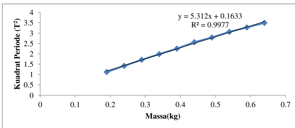
Gambar 9. Grafik hubungan antara massa dengan periode pegas 1
