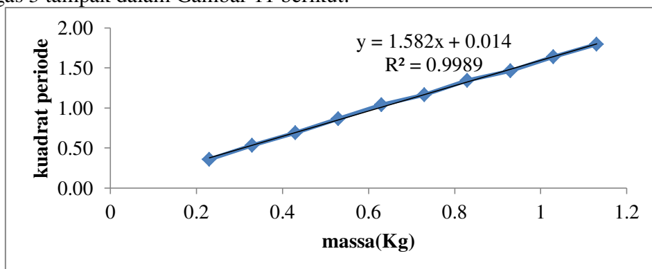
Gambar 11. Grafik hubungan antara massa dengan periode pegas 3
