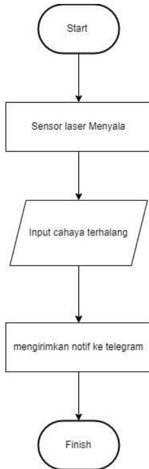
Gambar 4. Flowchart LDR dan laser sensor
