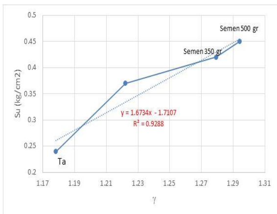
Gambar 12. Korelasi Kuat Geser Tanah (Su) Dengan Berat Volume ( \gamma ) Tanah Gambut Bercampur Semen dan Ecocure 21
