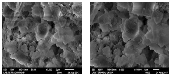
Gambar 6. SEM benda uji tanah gambut ditambah semen + Ecocure 21 dengan perbesaran 7500x dan 10000x
