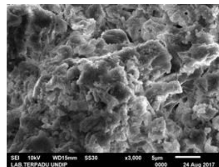
Gambar 4. SEM benda uji tanah gambut asli
