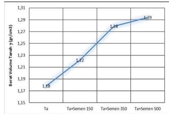
Gambar 7. Berat Volume ( \gamma ) Tanah Gambut Bercampur Semen
