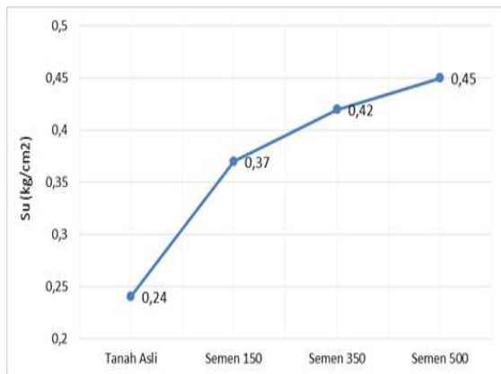
Gambar 9. Kuat Geser (Su) Tanah Gambut Bercampur Semen
