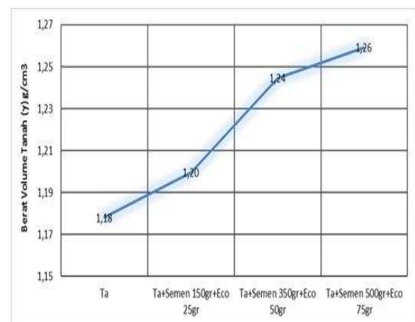
Gambar 8. Berat Volume ( \gamma ) Tanah Gambut Bercampur Semen dan Ecocure 21
