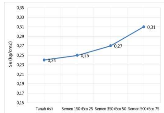
Gambar 10. Kuat Geser (Su) Tanah Gambut Bercampur Semen dan Ecocure 21
