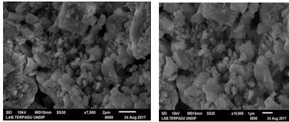
Gambar 5. SEM benda uji tanah gambut ditambah semen dengan perbesaran 7500x dan 10000x
