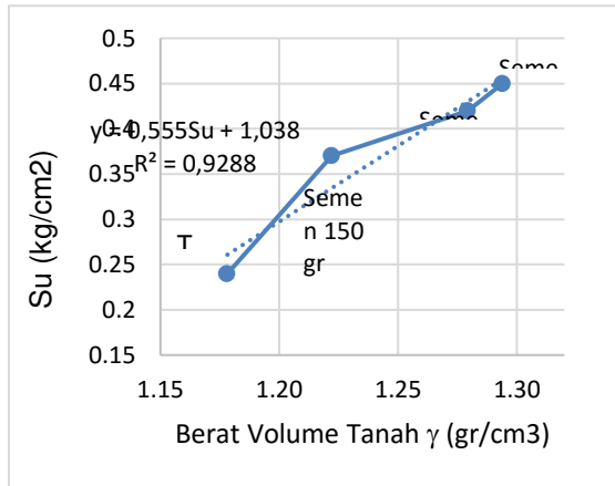
Gambar 11. Korelasi Kuat Geser Tanah (Su) Dengan Berat Volume ( \gamma ) Tanah Bercampur Semen
