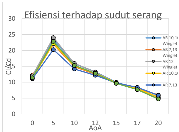
Gambar 13. Efisiensi pada setiap variasi sayap
