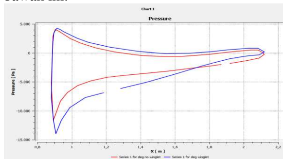
Gambar 14. Grafik distribusi tekanan
