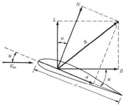
Gambar 1. Hubungan geometrik gaya aerodinamika [8]
