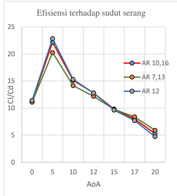
Gambar 8. Grafik efisiensi dari beragam variasi aspect ratio
