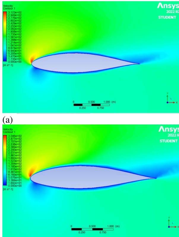
(a) (b) Gambar 7. Separasi aliran (a) AR 7,13 dan (b) AR 12
