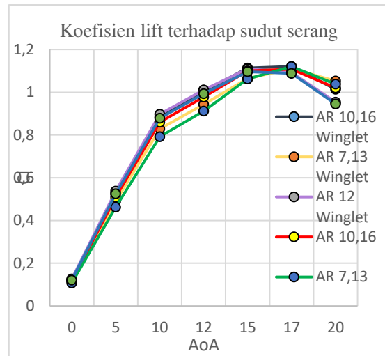
Gambar 10. Grafik Cl pada semua variasi sayap
