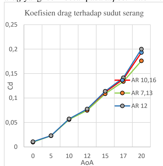
Gambar 6. Grafik C_d pada variasi aspect ratio
