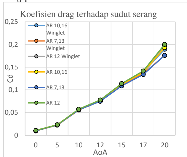
Gambar 12. Grafik Cd pada semua variasi sayap
