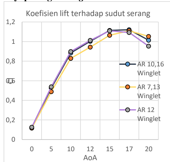
Gambar 9. Grafik Cl variasi sayap dengan winglet
