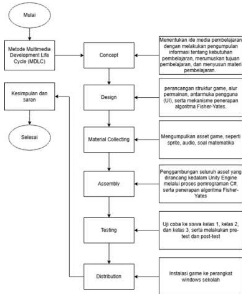
Gambar 1. Kerangka berpikir
