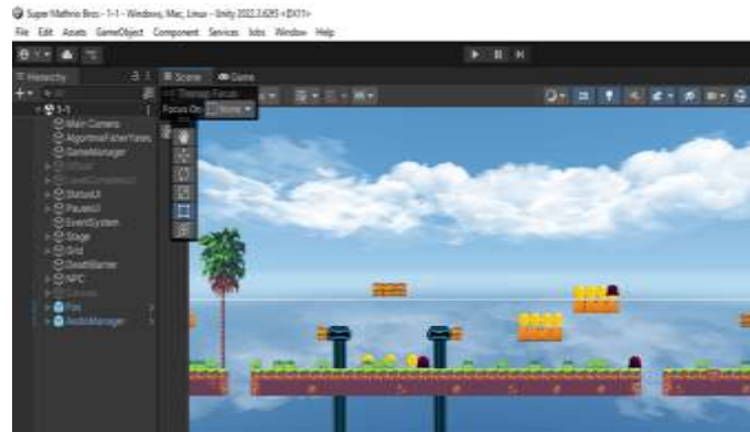
Gambar 5. Pembuatan scene
