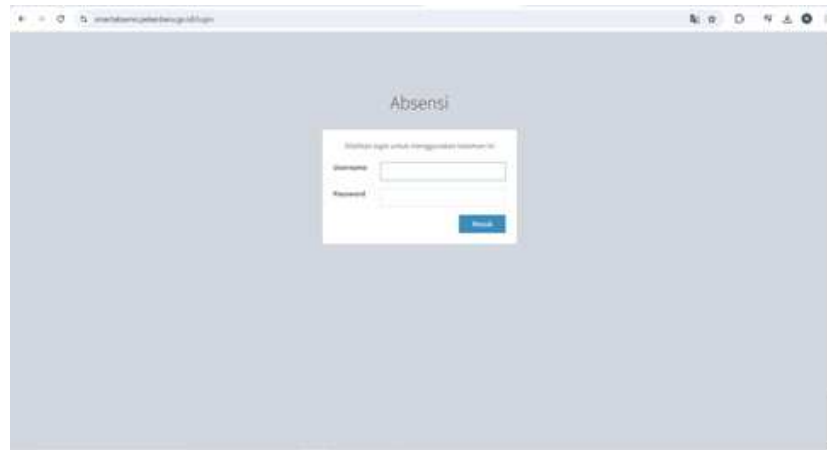
Gambar 5. Tampilan Login
