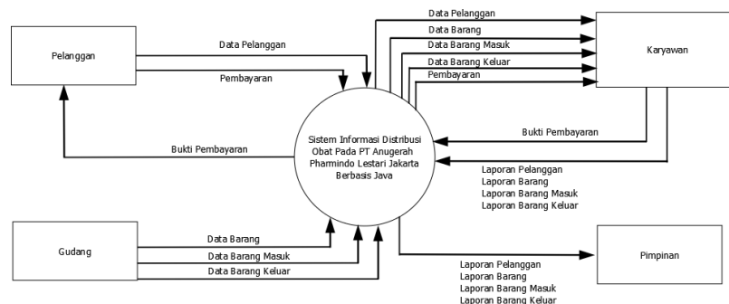
Gambar 2. Diagram Konteks Sistem
