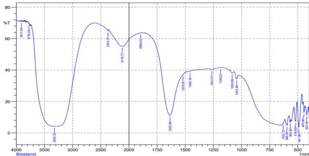
Gambar 4 Uji FTIR
