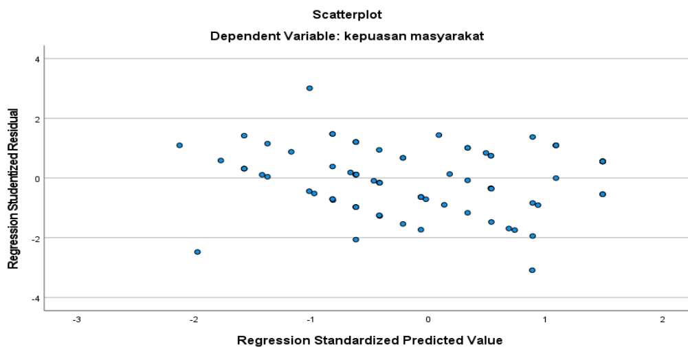
Gambar 3. Uji Heteroskedastisitas
