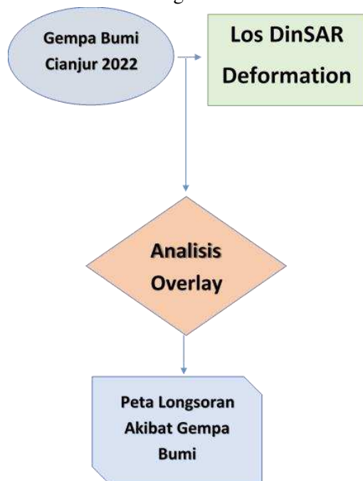
Gambar 1. Skema Penelitian
