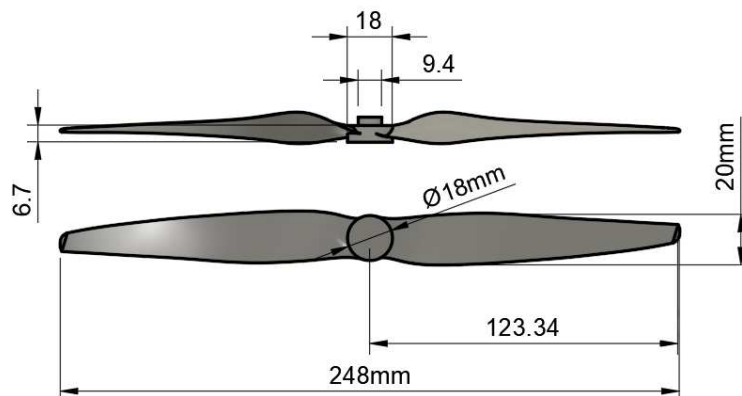
Gambar 3. Dimensi Propeler
