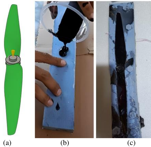
Gambar 10. Proses Penuangan Resin (a) Simulasi, (b) aktual, dan (c) hasil cetakan
