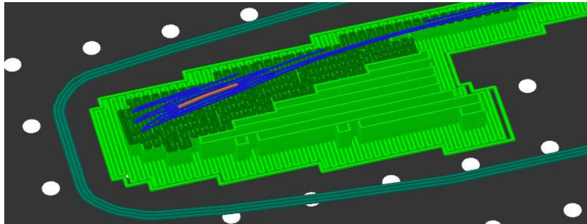
Gambar 16. Spacing support sebelum modifikasi
