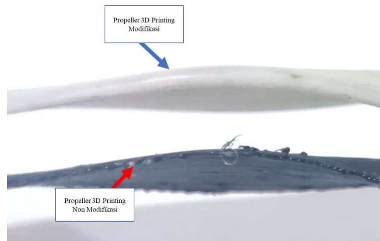
Gambar 18. Komparasi ketebalan antara propeler 3D printing modifikasi dan non-modifikasi
