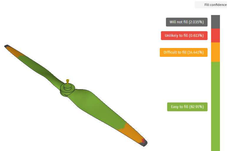
Gambar 11. Hasil simulasi persebaran resin
