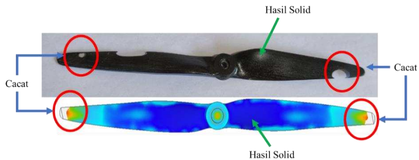
Gambar 13. Perbandingan hasil cetak resin dan simulasi sebelum optimasi
